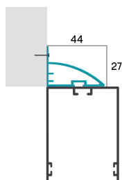
Front Fix aletta esterna
