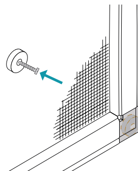
ATTACCO CON ANGOLO MAGNETICO IN APPOGGIO SU SUPERFICIE
